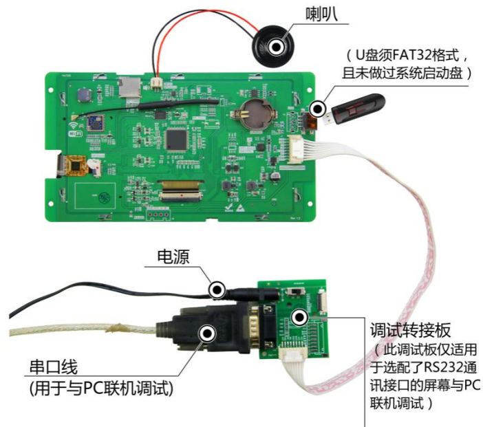
图 1-5 调试工具
